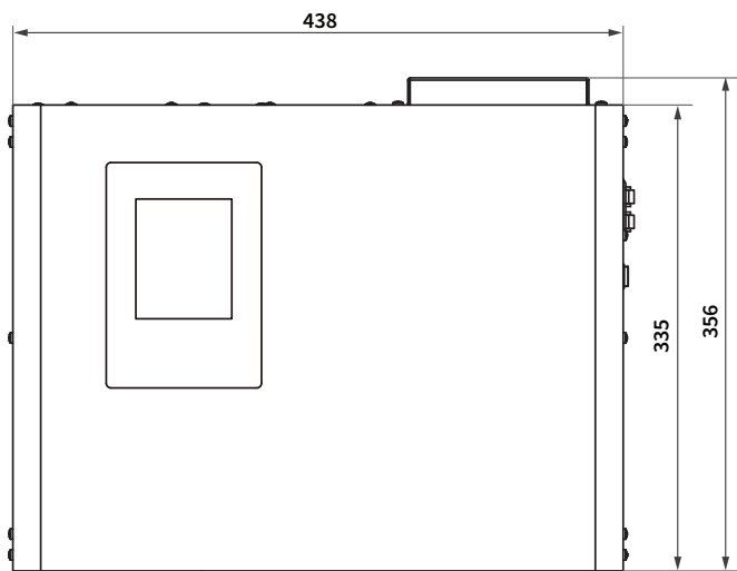
Voltek TCH-5 кВт
